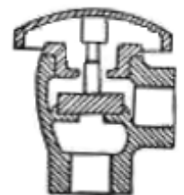
Sección transversal del AVB
