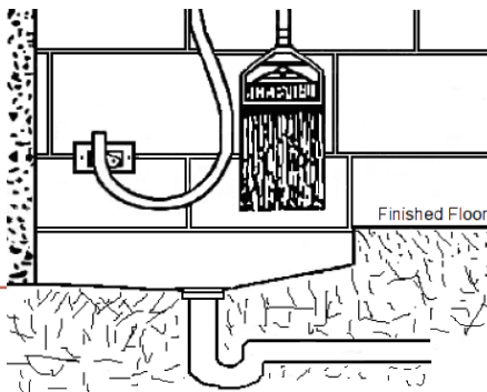
Fregadero de trapeador (lavabo empotrado)
