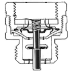
Sección transversal del grifo de manguera
