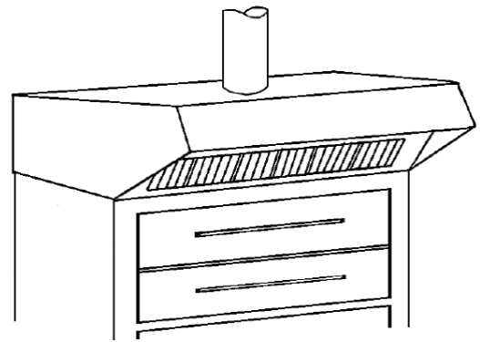
Campana de ceja (Montada en horno de pisos)
