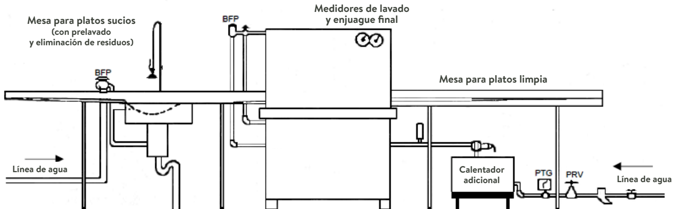
Ejemplo de instalación de una lavavajillas a máquina (unidad de desinfección con agua caliente) BFP = Dispositivo antirretorno PRV = Válvula reductora de presión PTG = Manómetro de presión y temperatura
