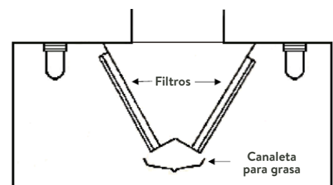
Campana de isla única (con un banco en V)
